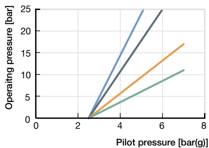
Actuator size: Ø130(P)
